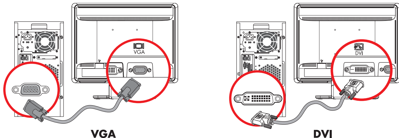
VGAまたはDVI-Dケーブルの接続 : コネクタの位置は異なる場合があります
