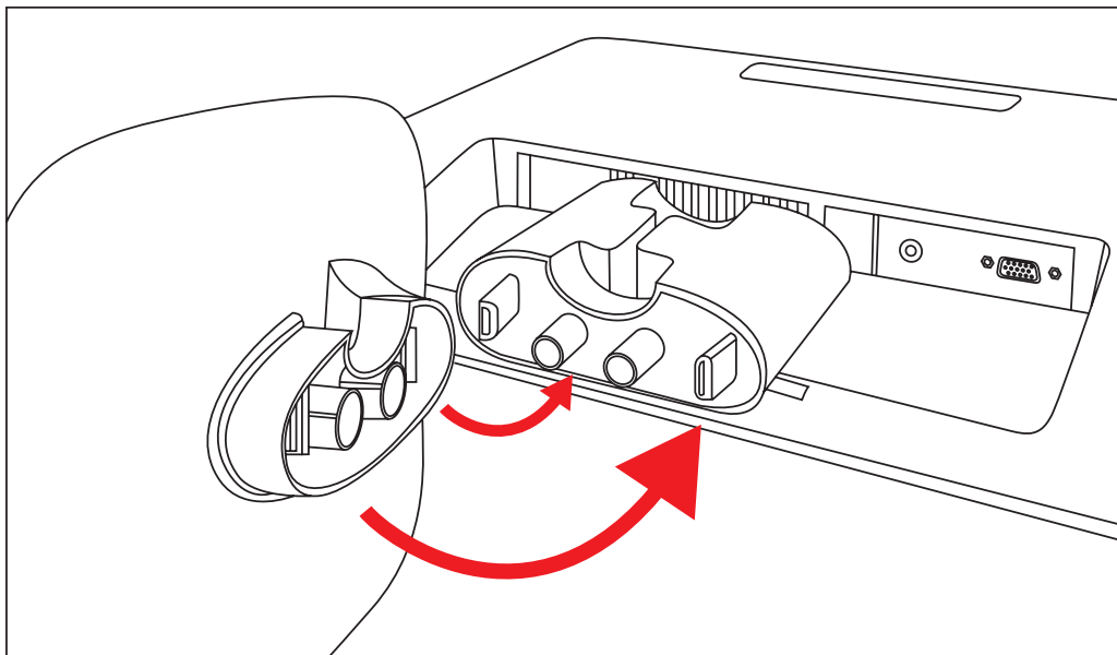
安裝顯示器底座
