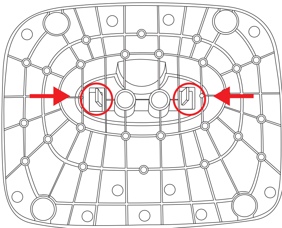
顯示釋放卡榫（圓圈部分）的顯示器底座底部示意圖
